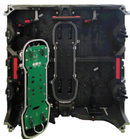
Power box completamente estraibile e sostituibile
